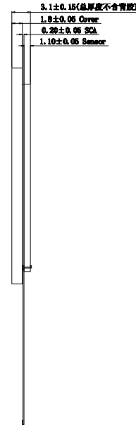
侧视图 横向10:1
