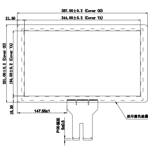
前视图 1:1
